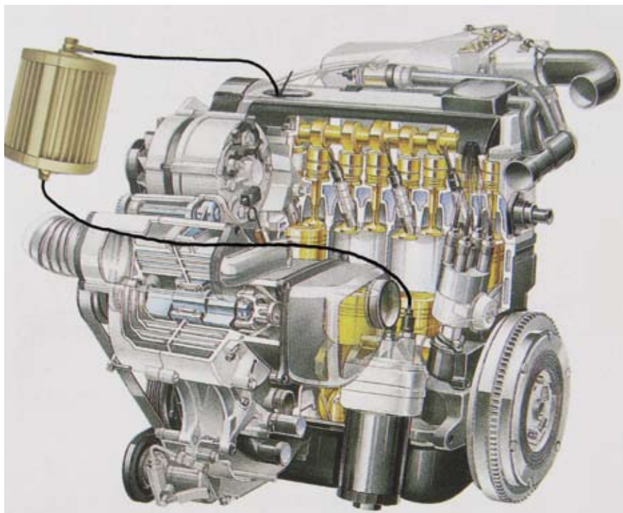
Prinzip des Nebenstromfilterprinzips: Die Öldruckabnahme erfolgt über ein T-Stück am Öldruckgeber, der Rücklauf über Ventildeckel/Einfüllstutzen.
